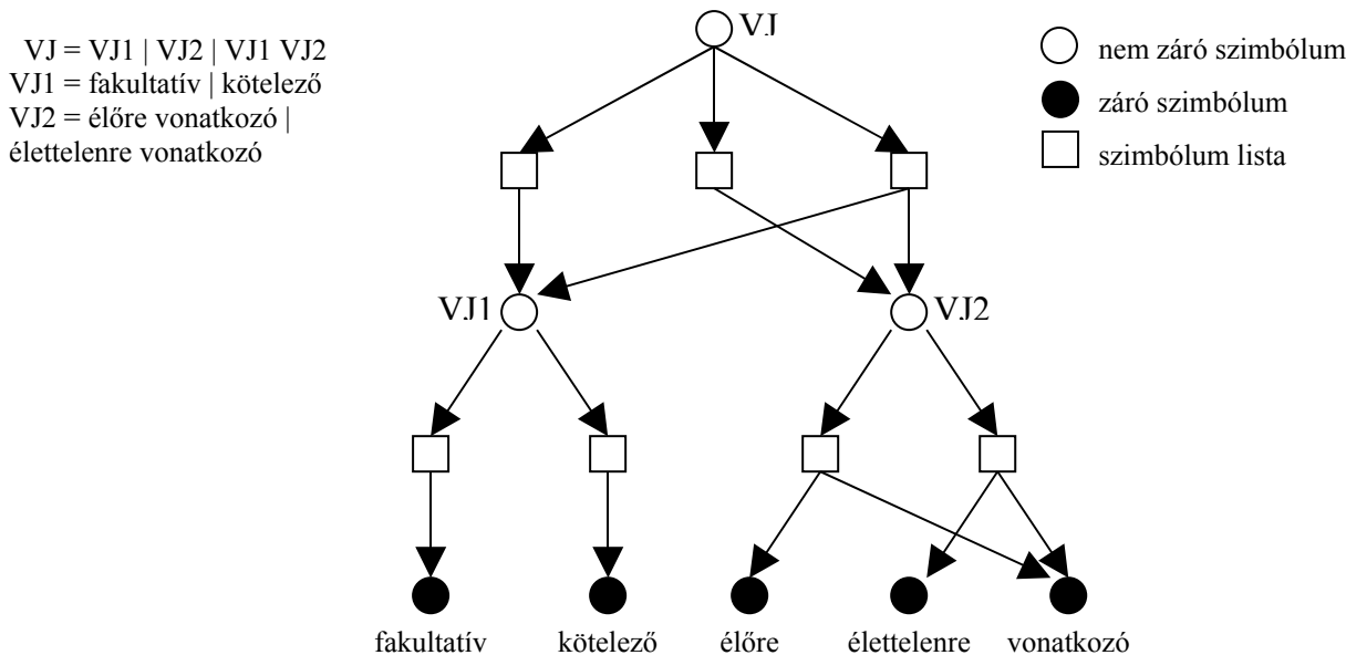
3. ábra: a vonatjelzők (VJ) reprezentációja tömörített erdővel
