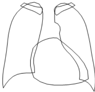
(d) b_2 = -3\sqrt{\lambda_2}
