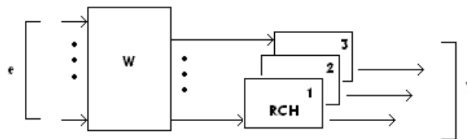
5.2. ábra. Többcsatornás zajcsökkentő rendszer blokkvázlata
