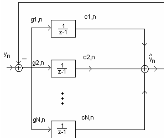
4.12. ábra. Rezonátoros megfigyelő integrátorokkal megvalósítva
