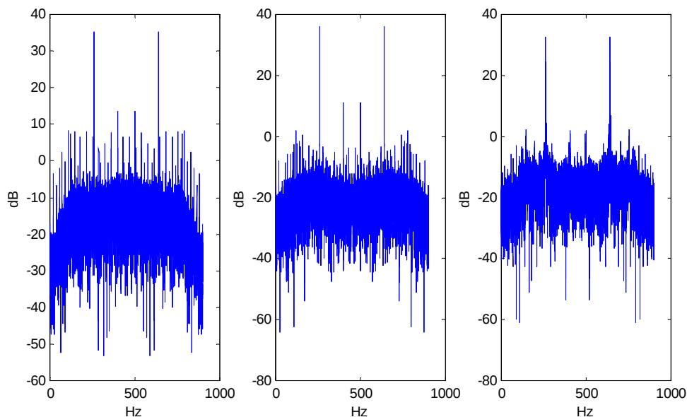
8.2. a,b,c ábra. Mintavételezett 260 Hz-es szinuszjel, f_s = 900 Hz
