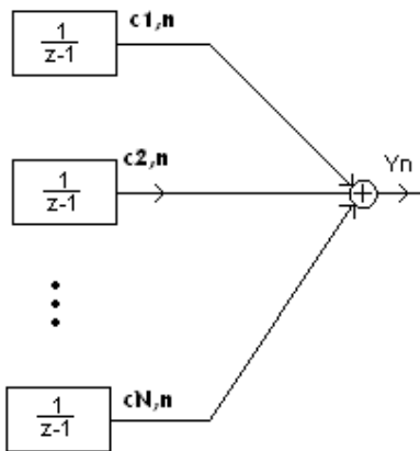
4.8. ábra. Sávkorlátozott periodikus jel modellje
