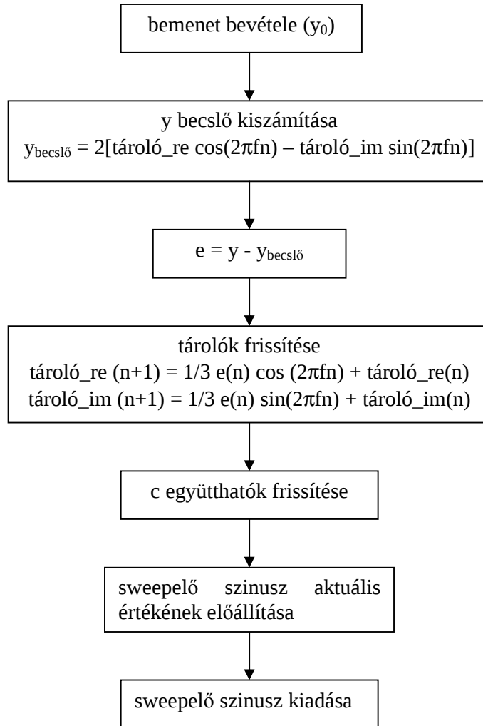
11.1. ábra. Az átviteli függvény mérő program folyamatábrája
