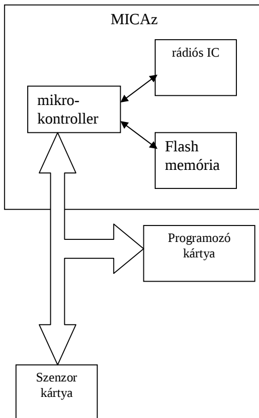
3.1 ábra. A MICAz mote-ok felépítése
