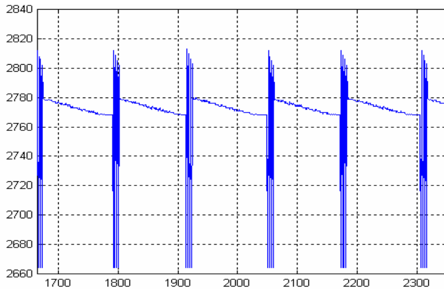
9.10. ábra. Rosszul beállított szabályzó
