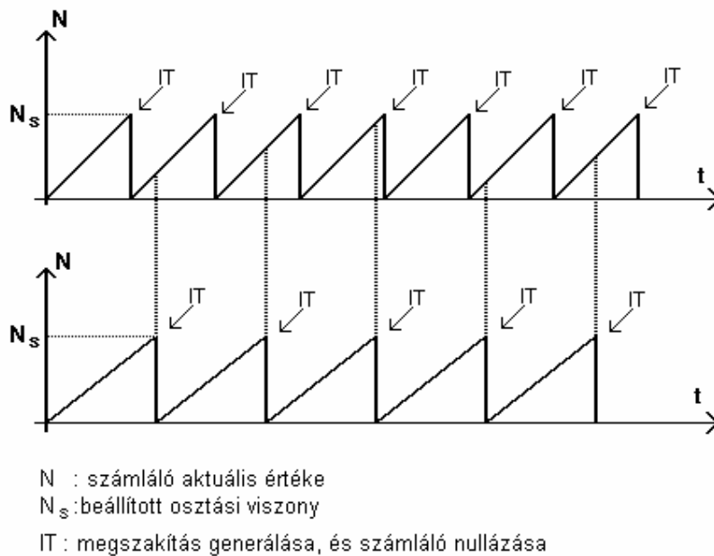
9.4. ábra. Az időzítő működése
