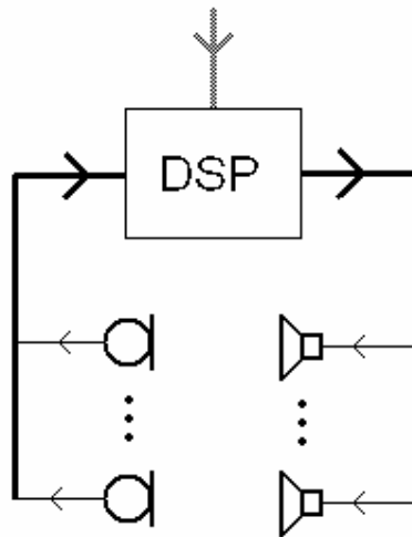
1.1. ábra. Egy aktív zajcsökkentő rendszer általános felépítése
