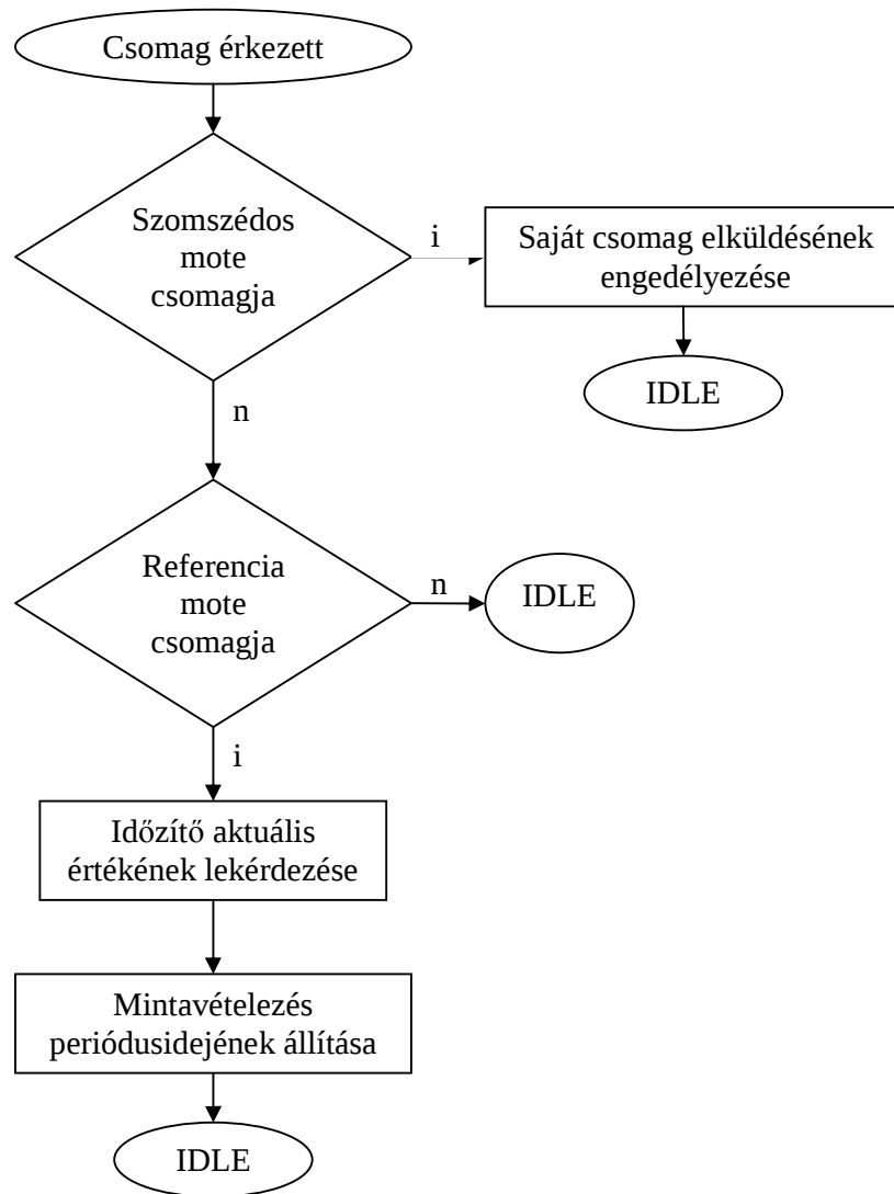
9.14. ábra. A hálózati működés időzítése és szinkronizálás
