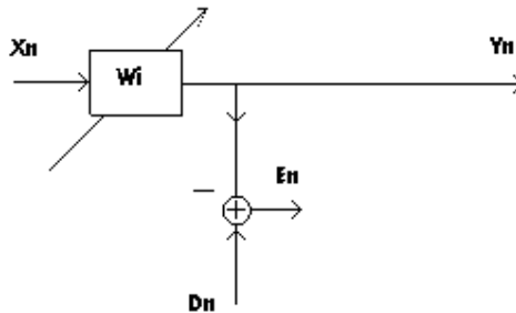
4.1. ábra. Az LMS algoritmus blokkvázlata
