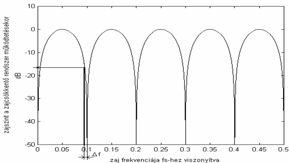
9.2. ábra. Zajcsökkentő rendszer átviteli függvénye
