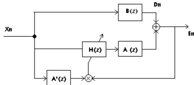
4.7. ábra. Az előrecsatolt rendszer blokkvázlata
