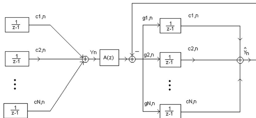
5.6. ábra. Átviteli függvény mérése rezonátoros struktúrával
