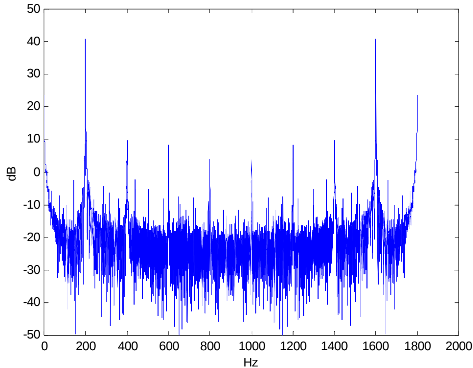
8.4. ábra. 200 Hz-es szinuszjel 1800 Hz-es mintavételi frekvenciával
