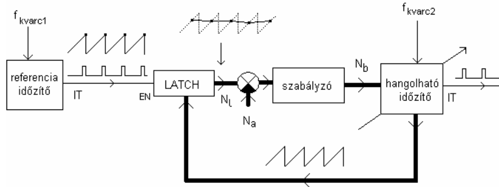
9.5.a. ábra. PLL analógia
