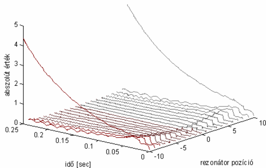
6.6. ábra. A hibajele Fourier-komponensekre bontó rezonátorkészlet rezonátorai abszolút értékének alakulása az idő függvényében, instabil rendszer esetén
