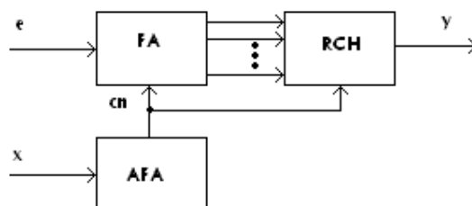
5.4. ábra. Megnövelt sebességű egycsatornás zajcsökkentő rendszer blokkvázlata
