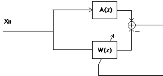
4.3. ábra. Átviteli függvény mérése LMS algoritmussal
