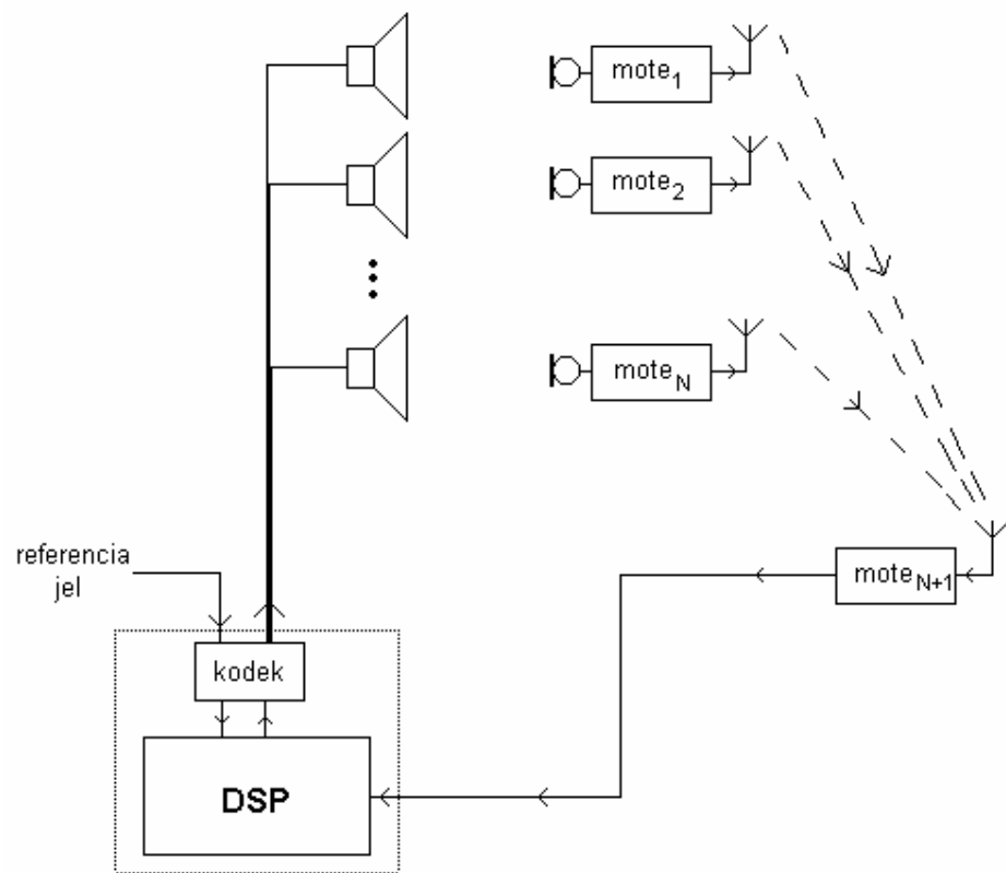
2.1. ábra. A zajcsökkentő rendszer tervezett felépítése
