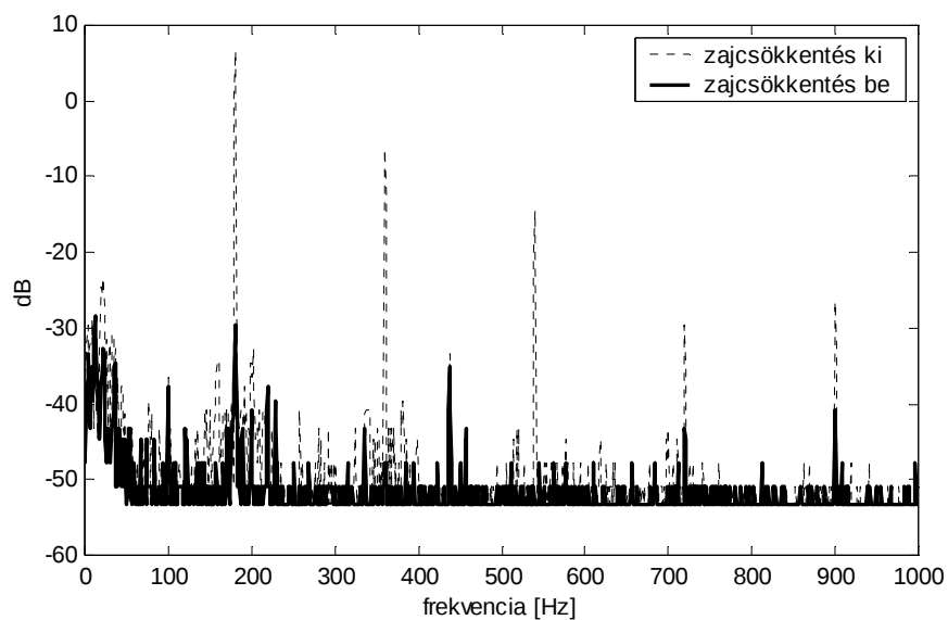
12.5. ábra. On-line identifikációs rendszer zajelnyomása állandósult állapotban az AFA referencia jele is rádión keresztül érkezik
