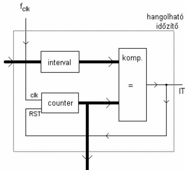
9.5.b. ábra. Hangolható időzítő
