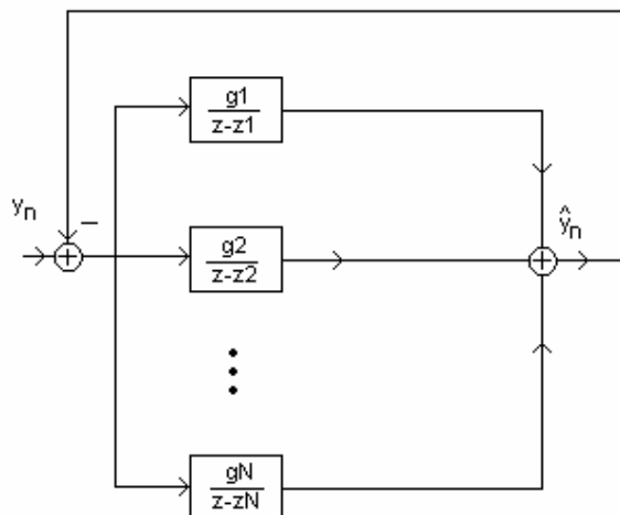
4.13. ábra. Rezonátoros megfigyelő rezonátorokkal megvalósítva
