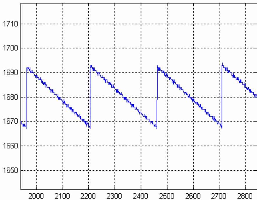
9.9. ábra. Helyesen beállított szabályzó állandósult állapotban
