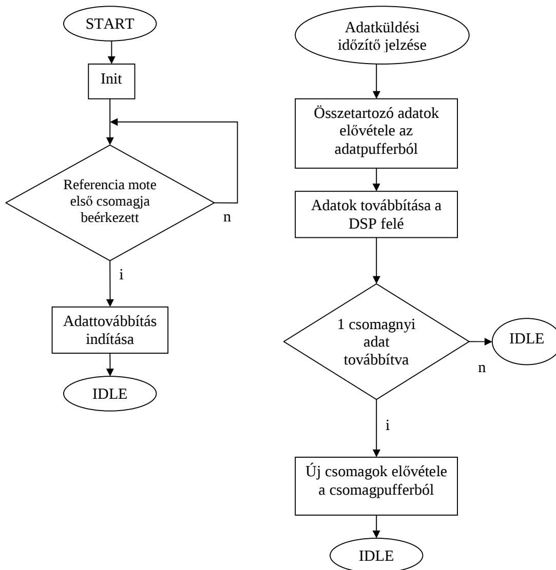
10.4. ábra. Inicializációs, és adattovábbítást vezérlő rész
