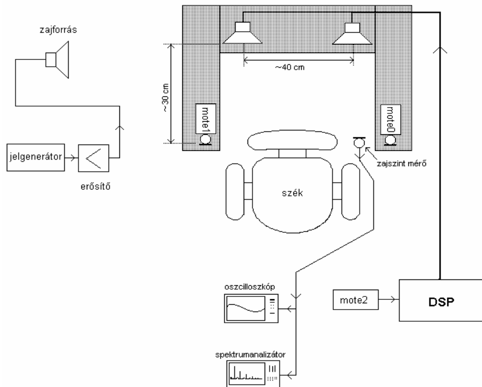
12.1. ábra. Zajelnyomó rendszer tesztkörnyezetének vázlata
