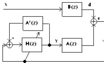
4.2. ábra. A visszacsatolt struktúra blokkvázlata
