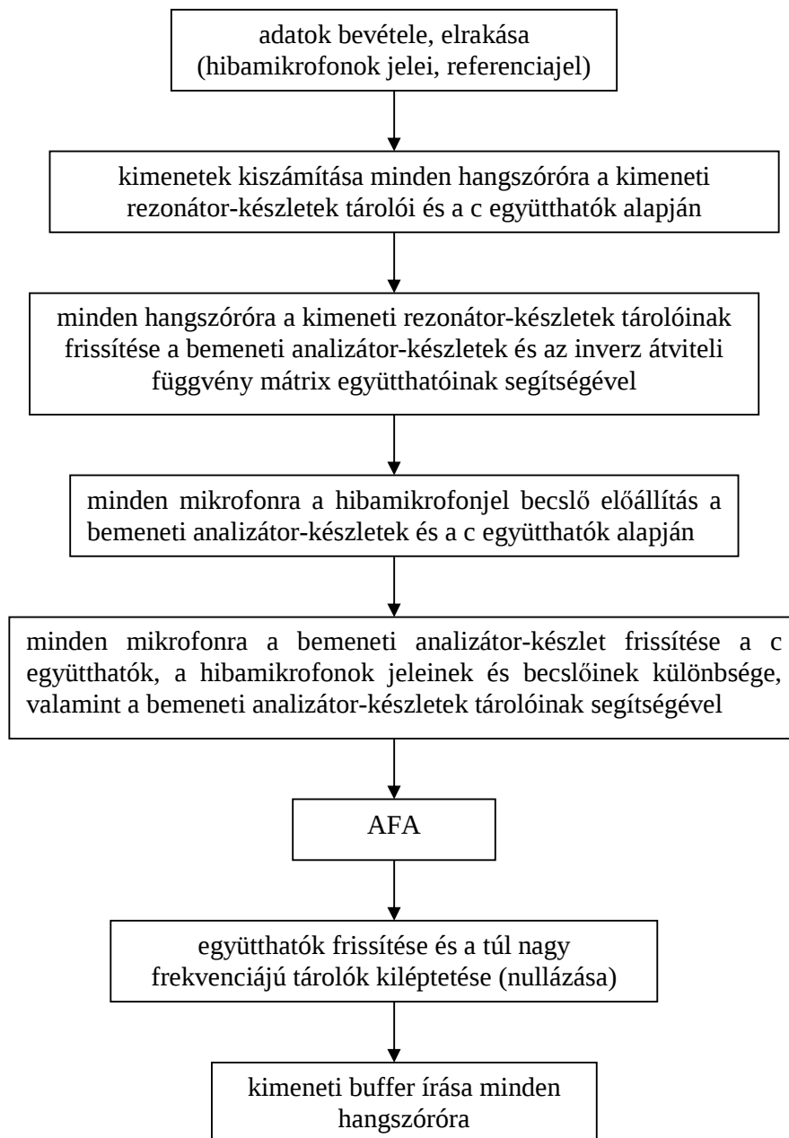
11.3. ábra. A többcsatornás zajcsökkentő program folyamatábrája
