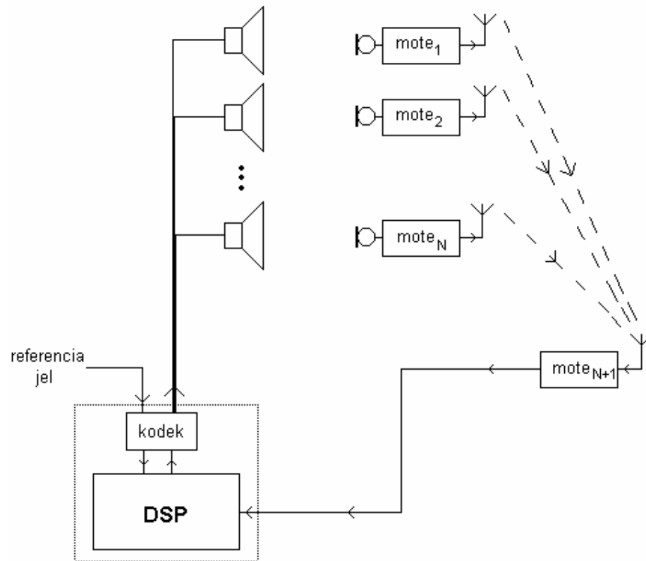
7.1. ábra. Rendszerterv
