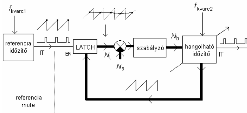
5.4. ábra. PLL analógia
