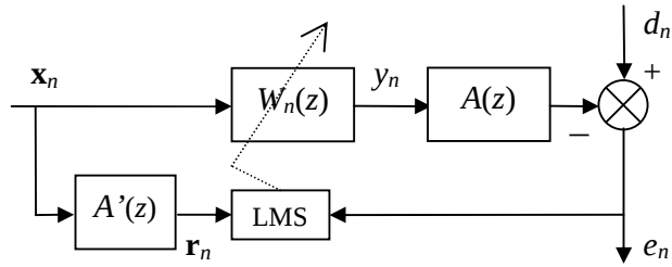
2.4. ábra. Előreccsatolt zajcsökkentő struktúra blokkvázlata
