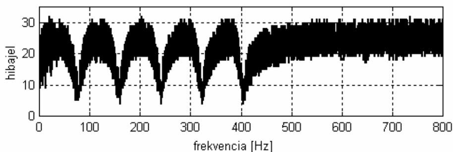
9.17. ábra. Hibajelre vonatkoztatott átvitel
