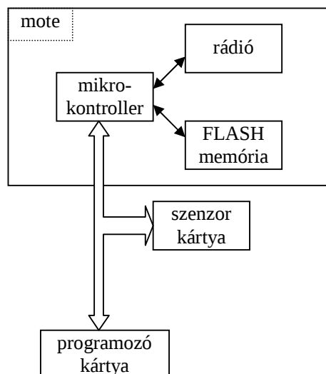
6.1. ábra. A MICAz mote-ok felépítése
