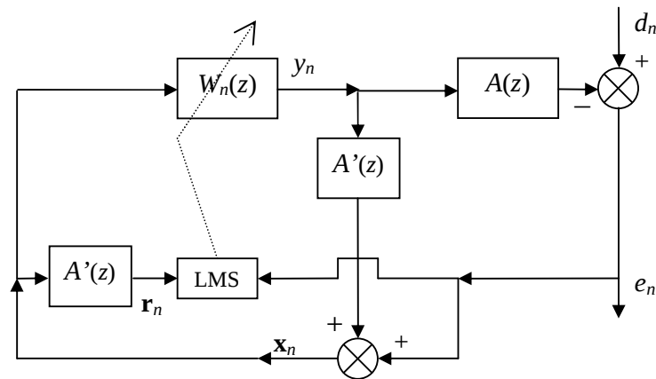
2.5. ábra. Viisszacsatolt zajcsökkentő struktúra
