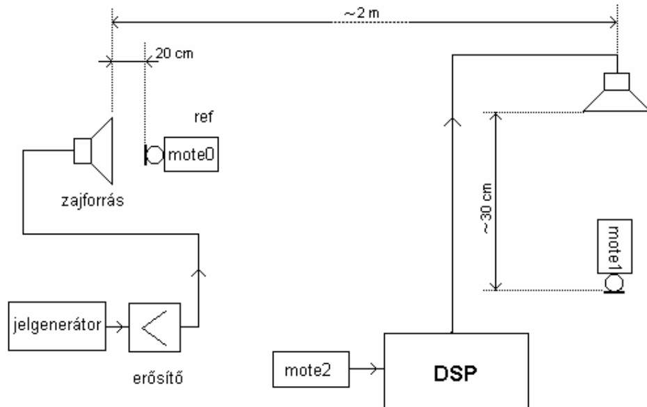
9.8. ábra. LMS alapú zajcsökkentő algoritmus tesztkörnyezete
