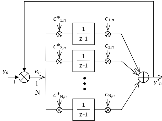
2.8. ábra. A koncepcionális jelmodellhez tartozó rezonátoros megfigyelő
