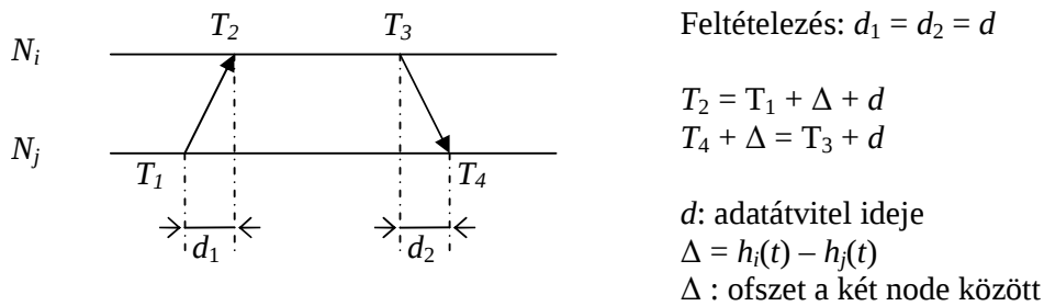
4.5. ábra. TEMPO algoritmus szemléltetése
