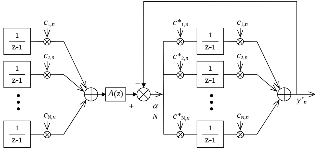
2.15. ábra. Identifikáció rezonátoros struktúrával
