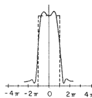
Köbös Spline
