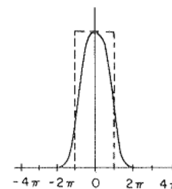
Köbös B-Spline
